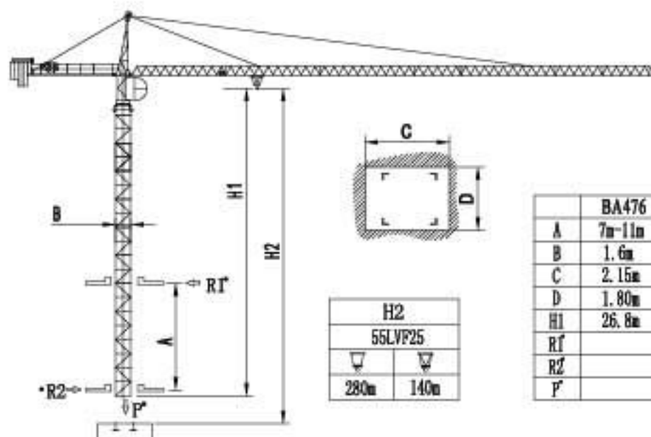
内爬塔机 Climbing crane
