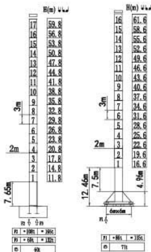
塔身截面 Mast 2.0mx2.0m
